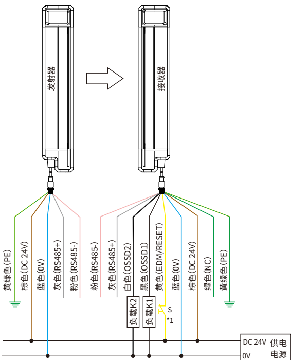
光同步：PNP输出接线图（无EDM、手动复位）
