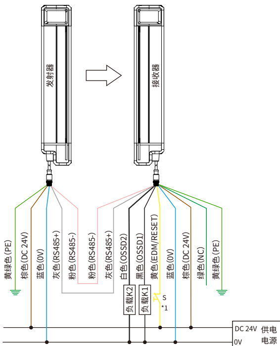
线同步：PNP输出接线图（无EDM、手动复位）
