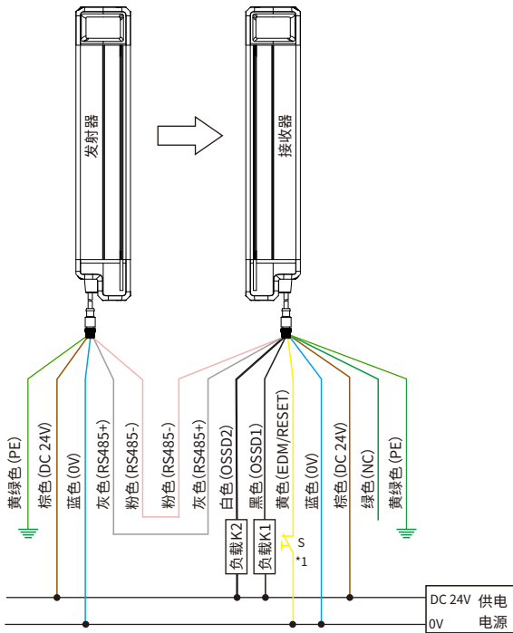
线同步：NPN输出接线图（无EDM、手动复位）
