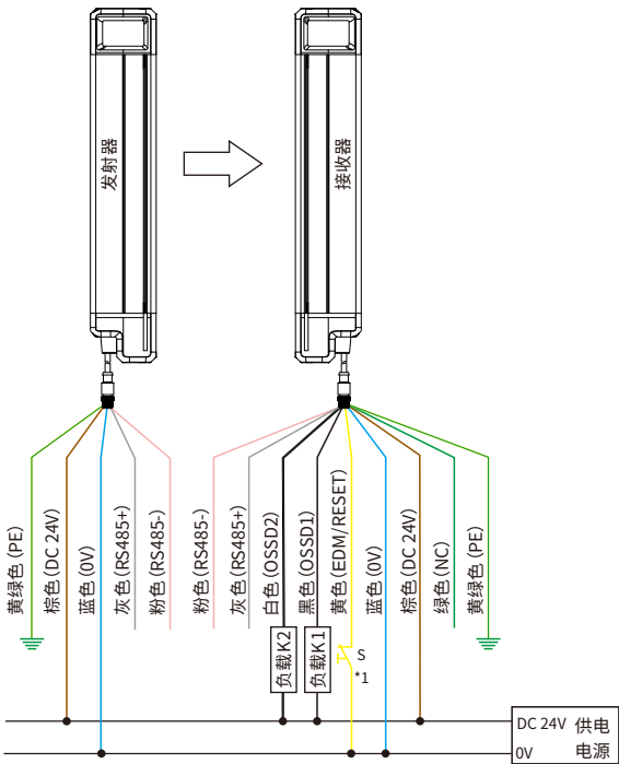
光同步：NPN输出接线图（无EDM、手动复位）
